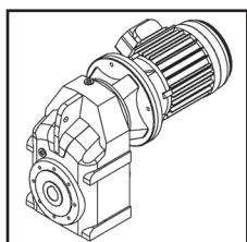
Серія F Плоскі циліндричні мотор-редуктори з паралельними валами
