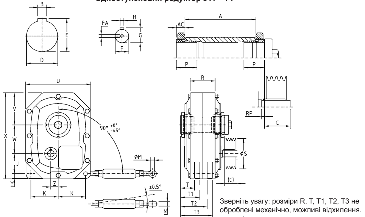
Одноступеневий редуктор J11 – 71
