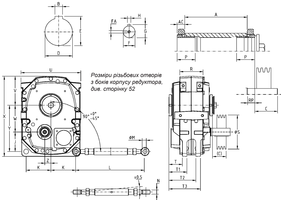
Одноступеневий редуктор J100 – 125
