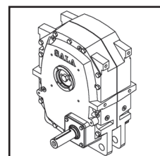
Серія J Циліндричні редуктори швидкості для монтажу на вал
