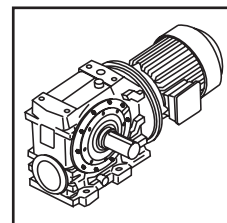
Серія С Циліндрично-черв'ячні мотор-редуктори та редуктори з перпендикулярними валами
