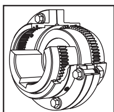
Зубчаста муфта серії X Жорстка на кручення високомоментна муфта
